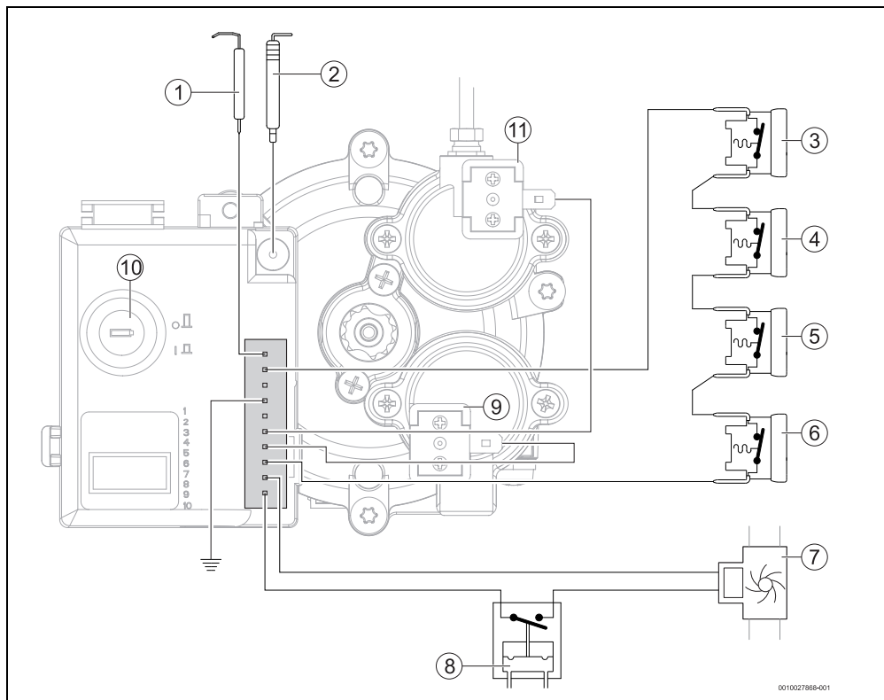
Joon. 24 Ühendusskeem
