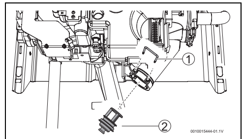
Joon. 9 Äravool
