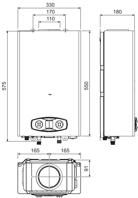
fig. 21 - Wymiary i podłączenia ZEFIRO ECO 11
