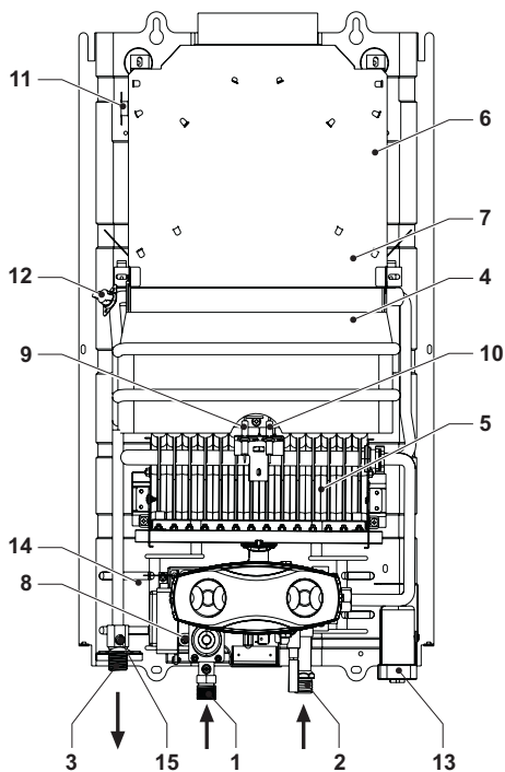
fig. 25 - Widok ogólny ZEFIRO ECO 14
