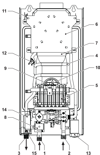
fig. 22 - Overview ZEFIRO ECO 6
