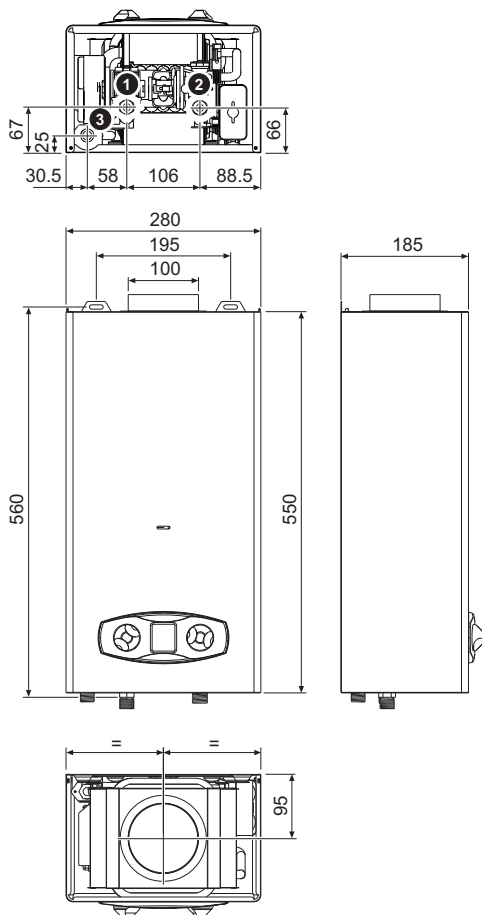
fig. 19 - Dimensioni e attacchi ZEFIRO ECO 6
