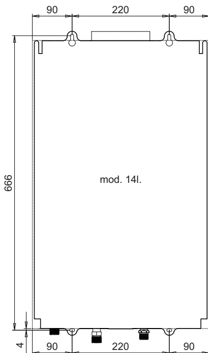
fig. 6 - Szablon montażowy
