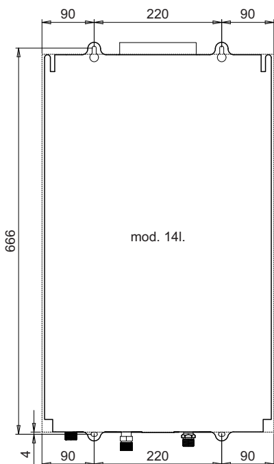
fig. 6 - Șablonul de montare
