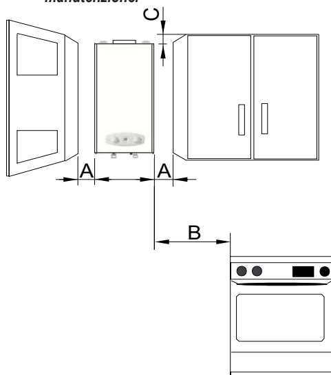
fig. 5 - Distanze minime
