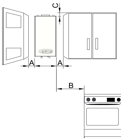
fig. 5 - Distanțe minime
