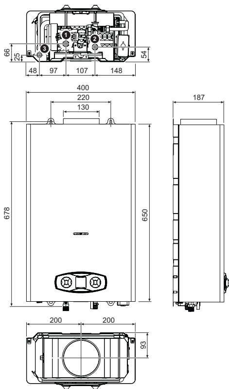
fig. 21 - Dimensioni e attacchi ZEFIRO ECO 14
