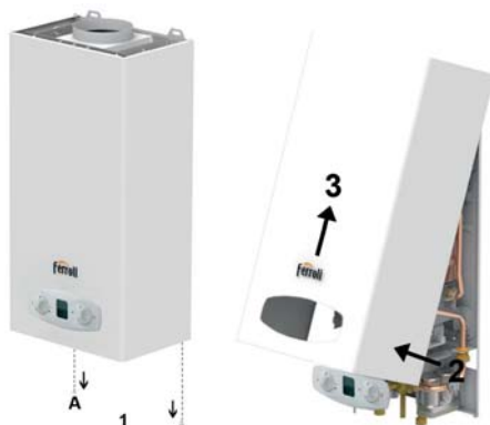
fig. 17 - Apertura del mantello
