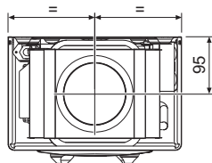
fig. 20 - Wymiary i podłączenia ZEFIRO ECO 6
