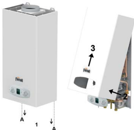
fig. 17 - Otwarcie obudowy
