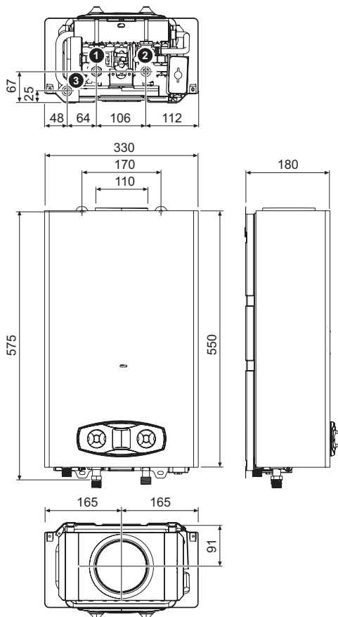
fig. 20 - Dimensiuni și racorduri ZEFIRO ECO 11
