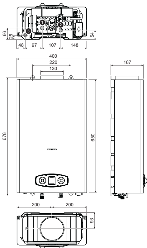
fig. 21 - Dimensiuni și racorduri ZEFIRO ECO 14
