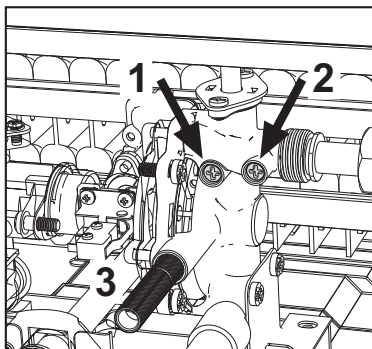
fig. 9 - śruby regulacji przepływu wody
