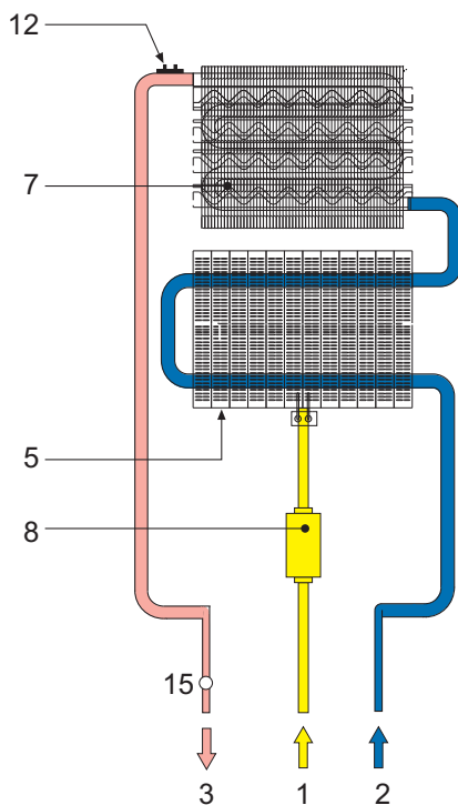
fig. 25 - Circuito idraulico
