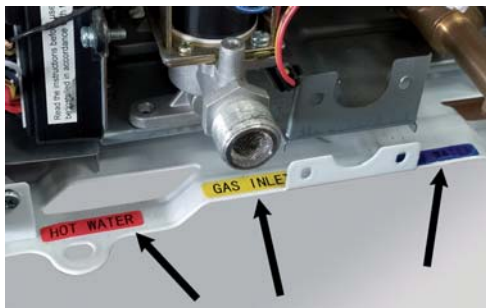
fig. 8 - Tabliczki informujące o podłączeniach
