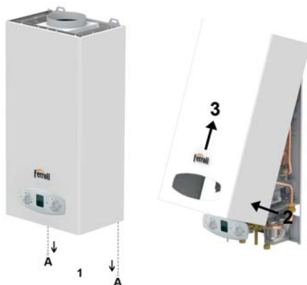
fig. 17 - Deschiderea carcasei
