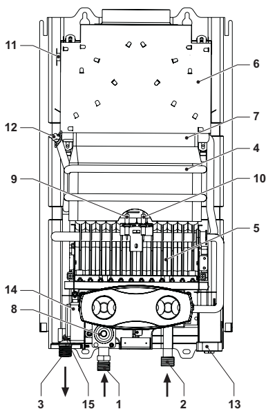
fig. 23 - Overview ZEFIRO ECO 11
