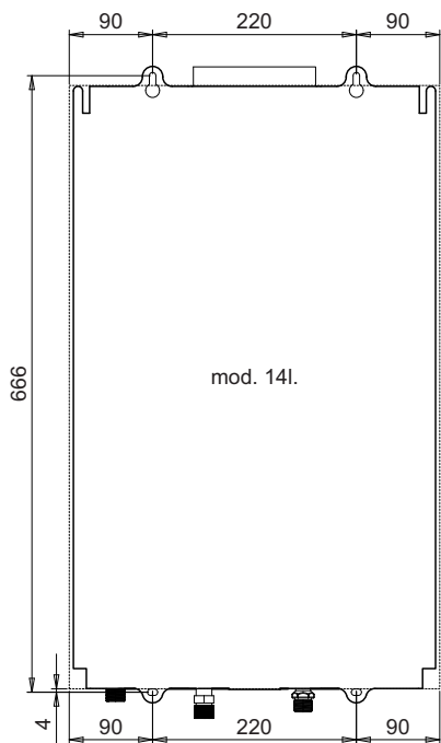
fig. 6 - Assembly template
