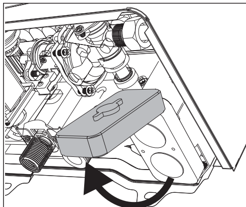
fig. 18 - Apertura dello scomparto delle batterie.
