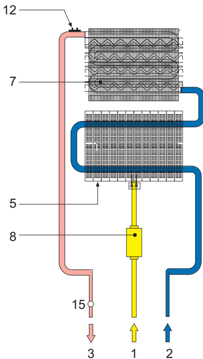
fig. 25 - Circuitul hidraulic
