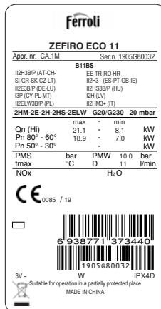
fig. 7 - Targhetta con le caratteristiche
