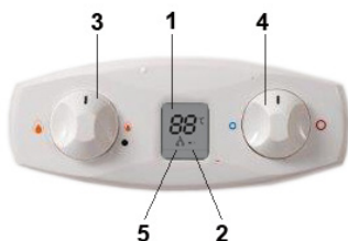
fig. 1 - Panoul de comandă
