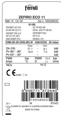
fig. 7 - Plăcuța cu datele tehnice
