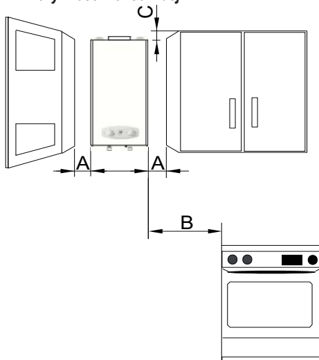
fig. 5 - Minimalne odległości
