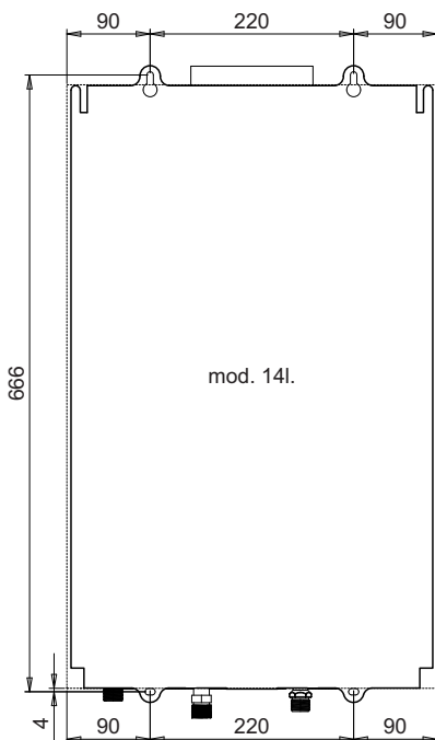
fig. 6 - Dima di montaggio
