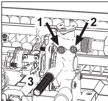
fig. 9 - Viti regolazione portata acqua
