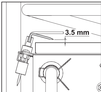
fig. 16 - Posizione elettrodo
