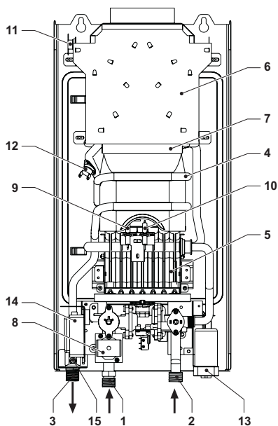
fig. 22 - Vista generale ZEFIRO ECO 6
