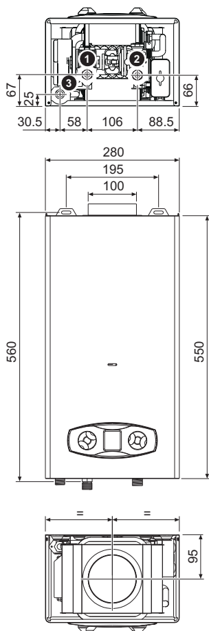
fig. 19 - Dimensiuni și racorduri ZEFIRO ECO 6
