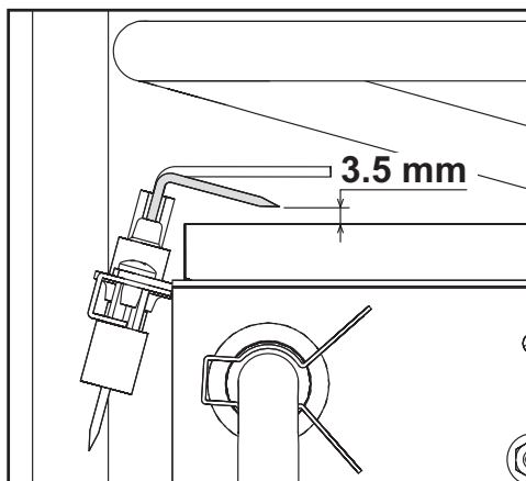
fig. 16 - Poziție electrozi
