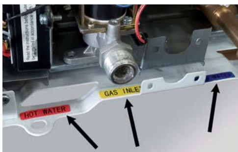
fig. 8 - Allacciamenti
