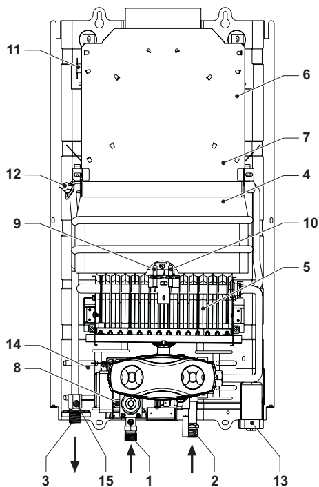
fig. 24 - Vista generale ZEFIRO ECO 14
