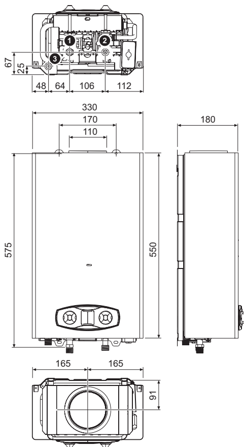
fig. 20 - Dimensioni e attacchi ZEFIRO ECO 11
