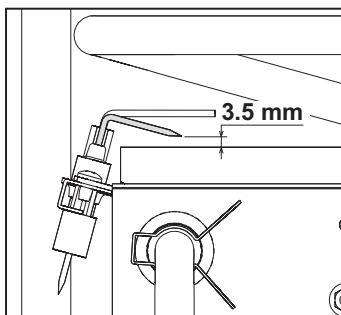
fig. 16 - Pozycja elektrod
