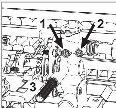
fig. 9 - Șuruburi de reglare a debitului de apă
