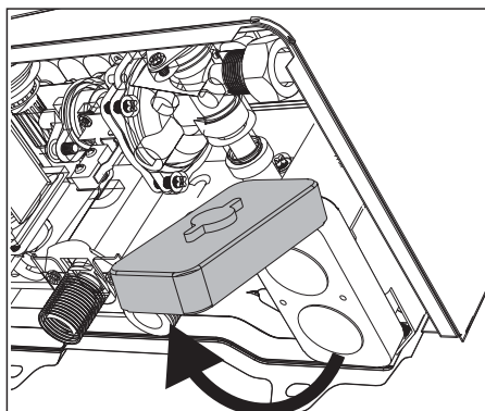
fig. 18 - Deschiderea compartimentului bateriilor.
