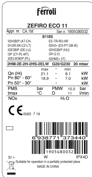
fig. 7 - Tabliczka znamionowa
